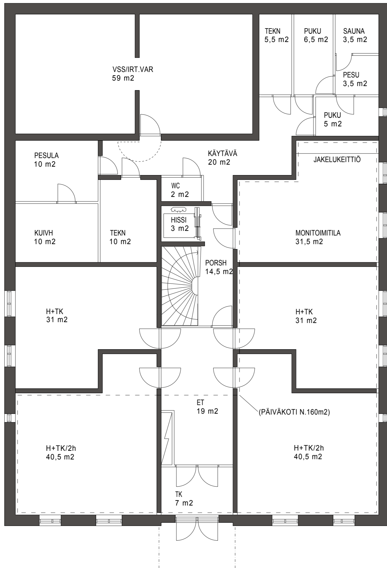
POHJAKAAVIO KELLARI 1:100
